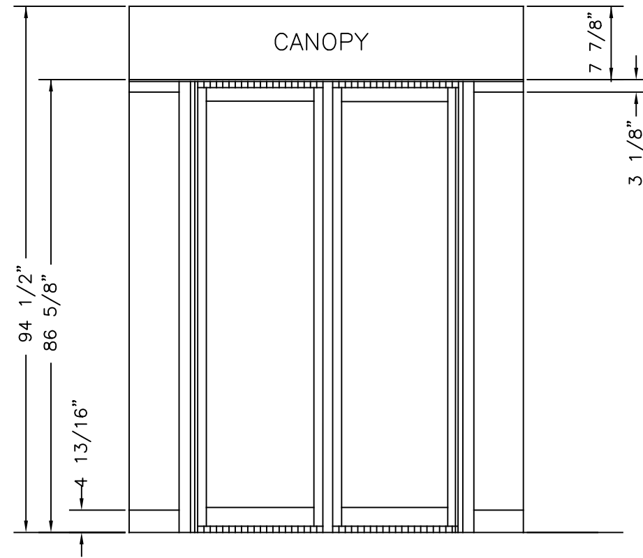
ELEVATION
